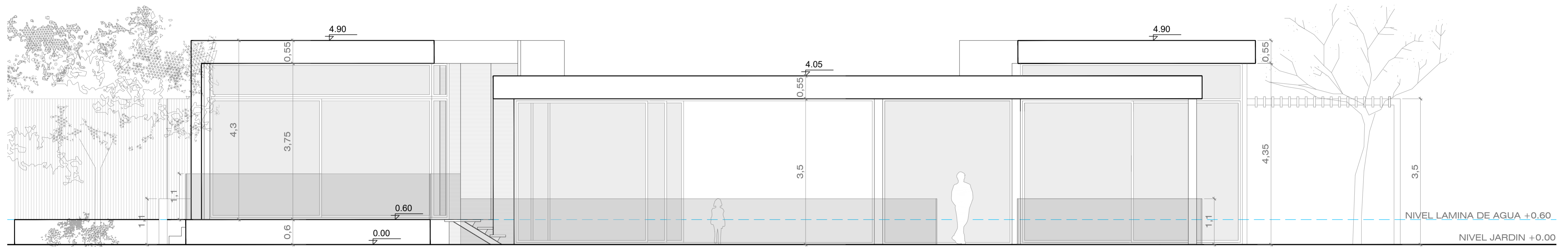
ALZADO 2
