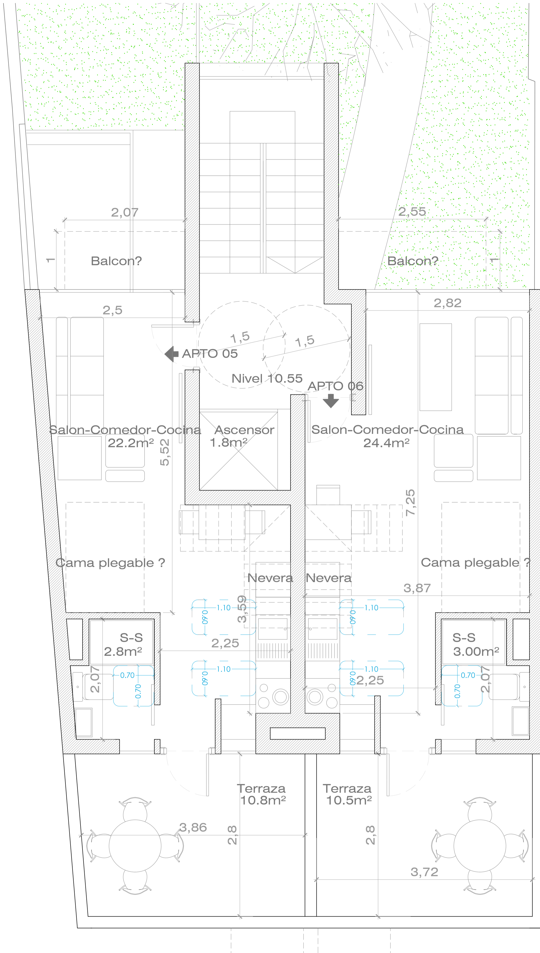
PLANO DE DISTRIBUCION PLANTA ATICO OPCION 05 SUPERFICIE CONSTRUIDA ATICO 05 28m 2 -SUPERFICIE UTIL 25m 2 SUPERFICIE CONSTRUIDA ATICO 06 32m 2 -SUPERFICIE UTIL 27.4m 2 SUPERFICIE CONSTRUIDA TOTAL PLANTA ATICO 74m 2 ESCALA: 1/75 AM Arquitectos
