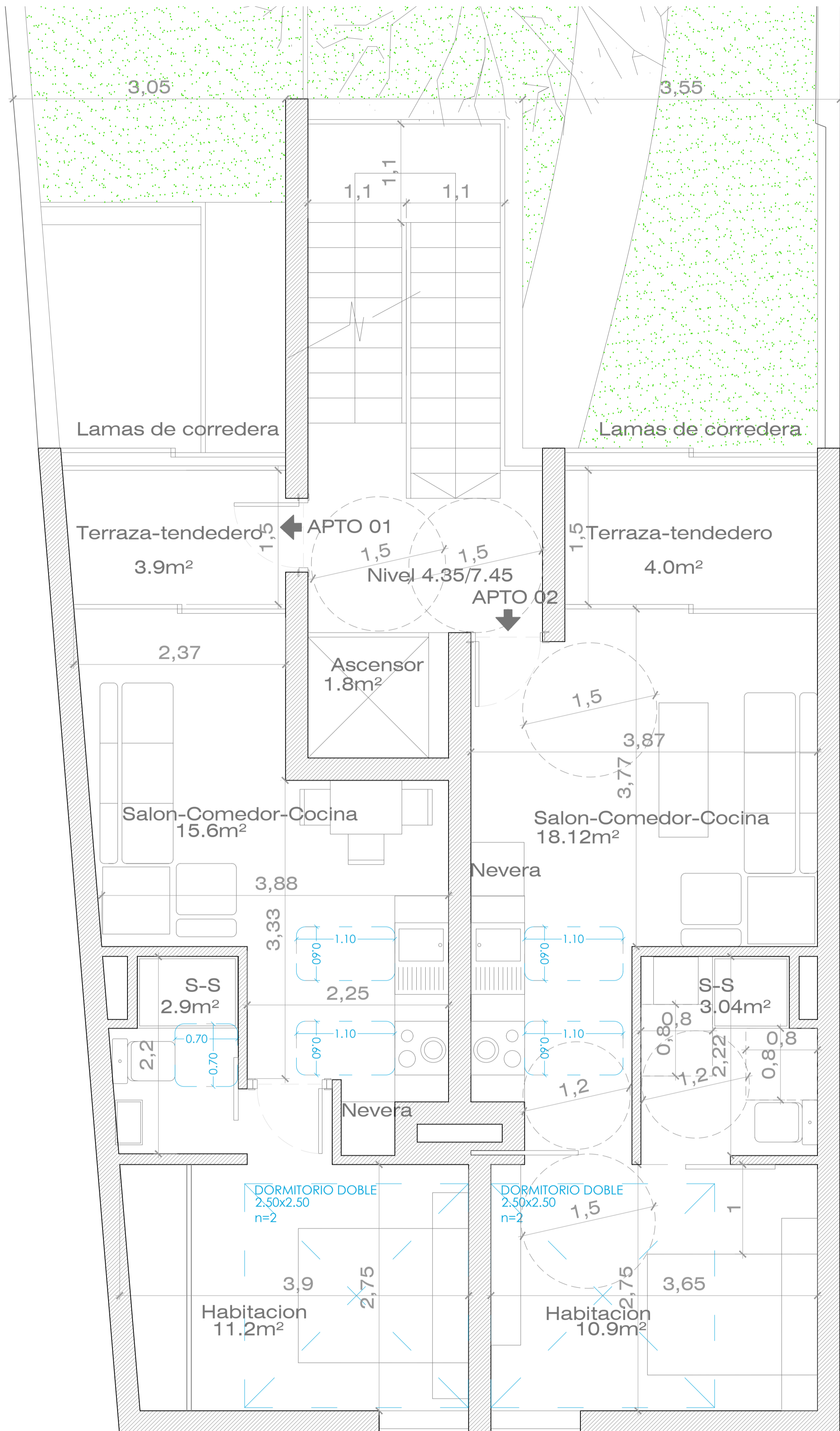
PLANO DE DISTRIBUCION PLANTA PRIMERA APARTAMENTOS 01 y 02 SUPERFICIE CONSTRUIDA APTO 01 34.5m 2 -SUPERFICIE UTIL 29.7m 2 SUPERFICIE CONSTRUIDA APTO 02 (ADAPTADO MINUSVALIDOS) 38.20m 2 -SUPERFICIE UTIL 32.06m 2 SUPERFICIE CONSTRUIDA TOTAL PLANTA PRIMERA 87m 2 ESCALA: 1/75 AM Arquitectos
