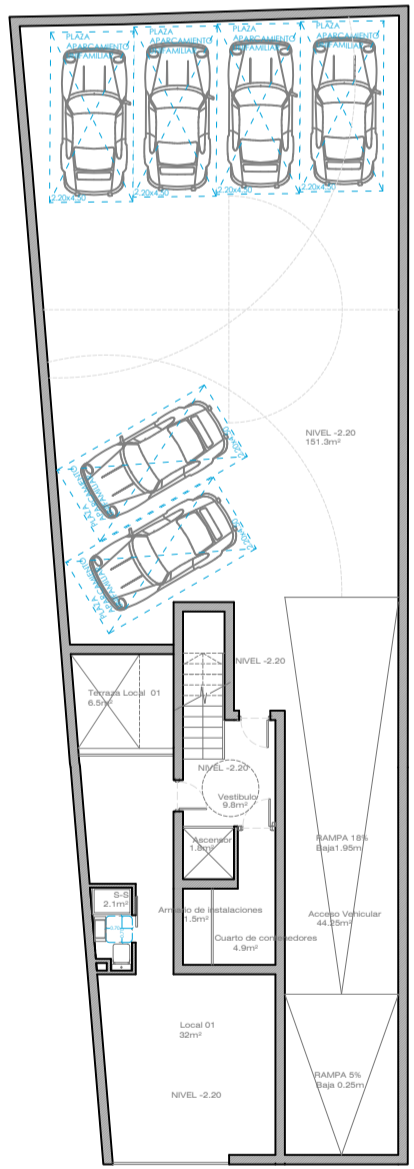
PROPUESTA DE APARCAMIENTO PLANTA SOTANO PLANO DE DISTRIBUCION PLANTA SOTANO + LOCAL 01 SUPERFICIE CONSTRUIDA PLANTA BAJA LOCAL 01 37.7m2 ESCALA: 1/75 AM Arquitectos
