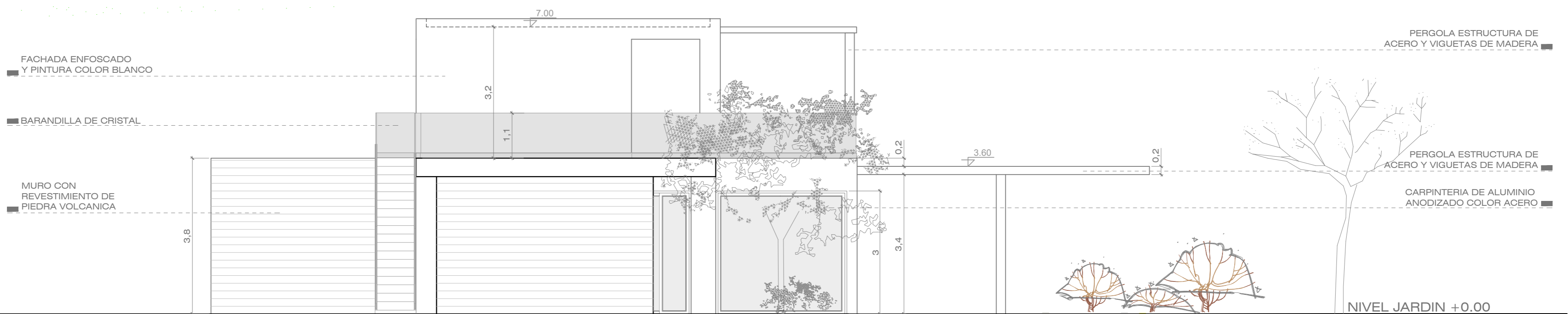
ALZADO LATERAL IZQUIERDO
