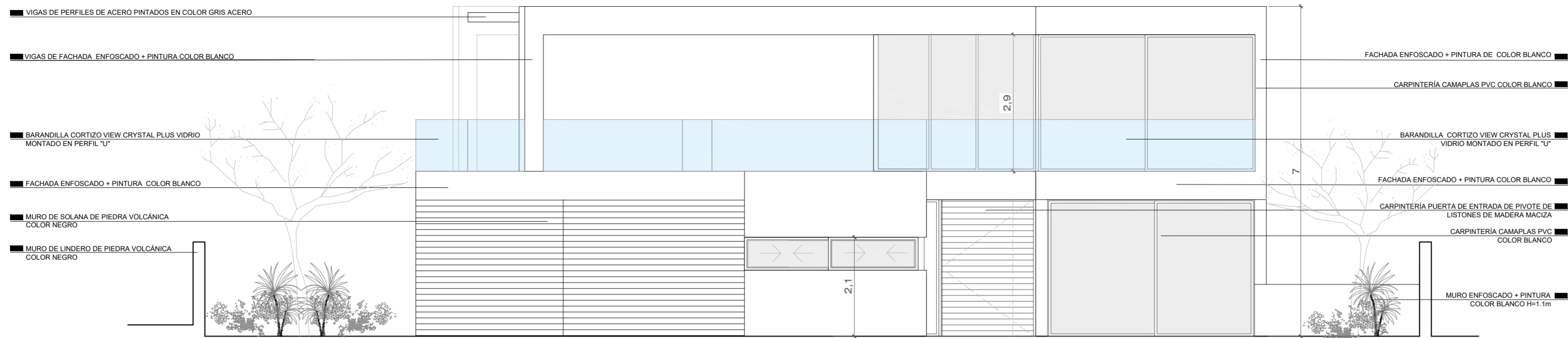
ALZADO NORTE CALLE ERIZO
