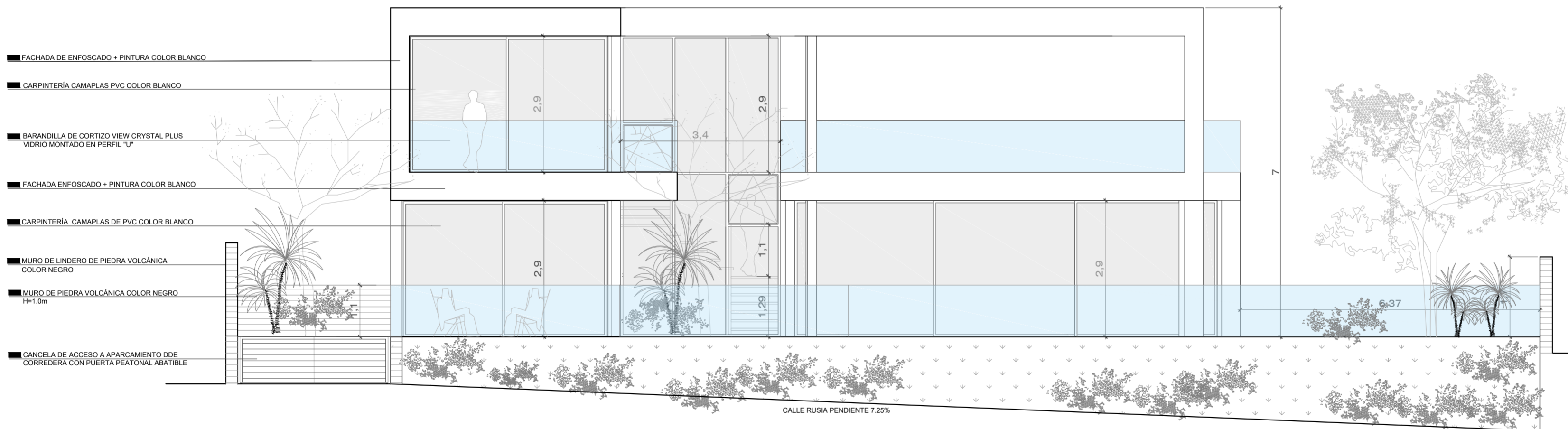
ALZADO SUR CALLE RUSIA
