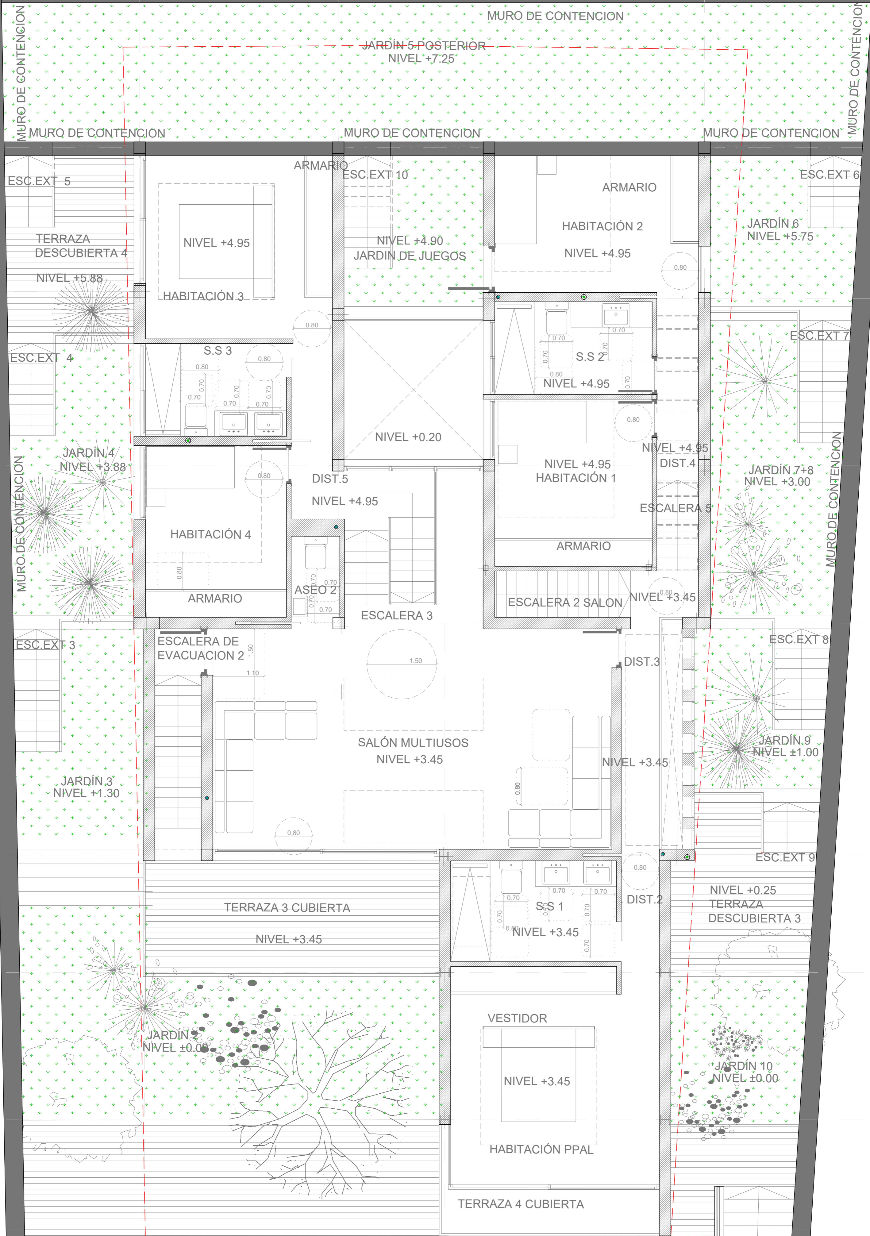
PLANO DE DISTRIBUCIÓN PLANTA PRIMERA. HABITABILIDAD VARIANTE 12
